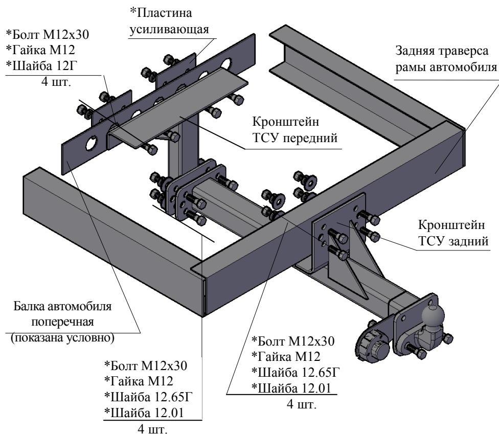
РИС.1 Тягово-сцепное устройство ТСУ 3163.K2
