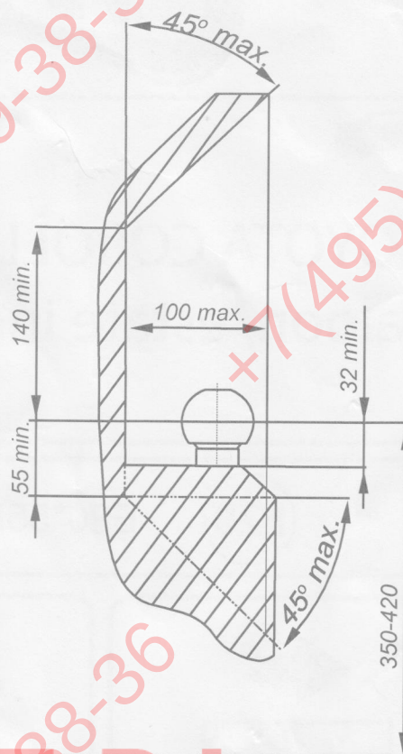
PRZĘKRÓJ A-A
