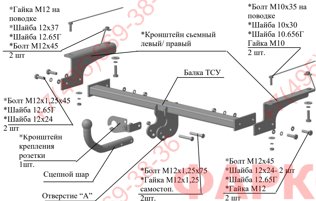
Рис.1 Тягово-сцепное устройство 8140
