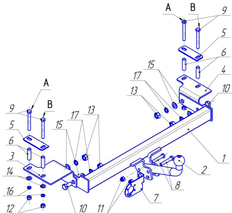
Рис.1 Установка на автомобиль
